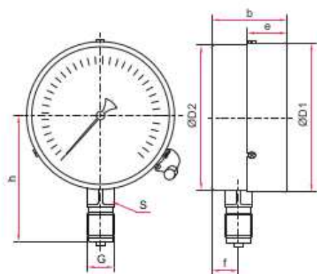
1. Радиальное присоединение
