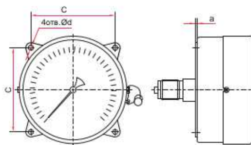
2. Осевое присоединение
