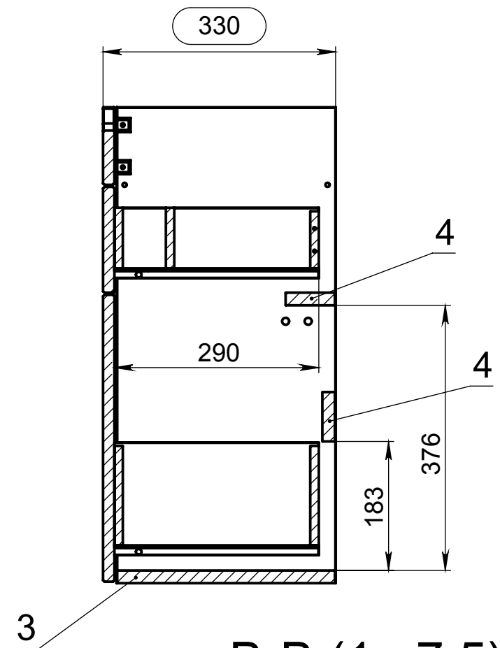
B-B (1 : 7.5)
