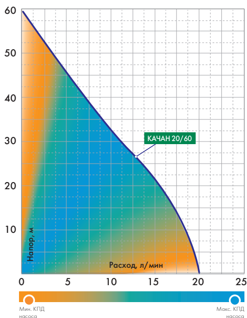
График расходно-напорных характеристик*
