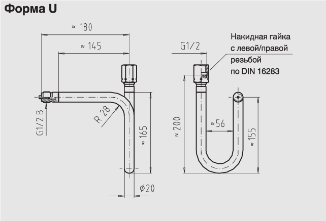
Сифон формы «виток»
