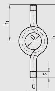
Сифон формы «виток»
