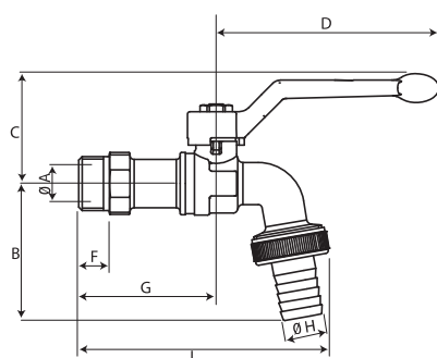
DN 15-20
