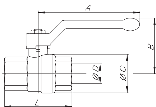
Габаритные и присоединительные размеры
